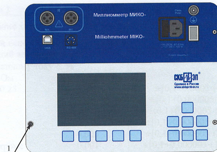
Рисунок 2 – Схема пломбировки от несанкционированного доступа 1 – место нанесения оттиска пломбы изготовителя
