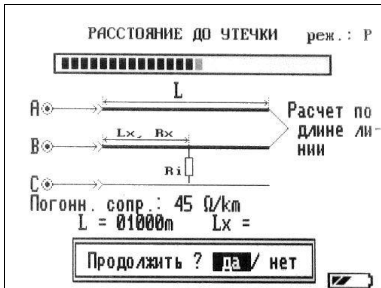
Рисунок 6-18 Метод Муррея
