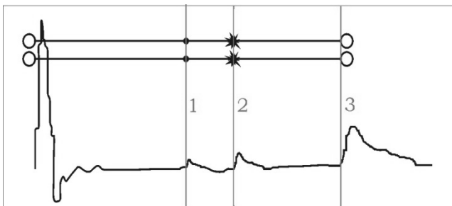
Рисунок 6-1 Муфты, скрутки, обрывы
