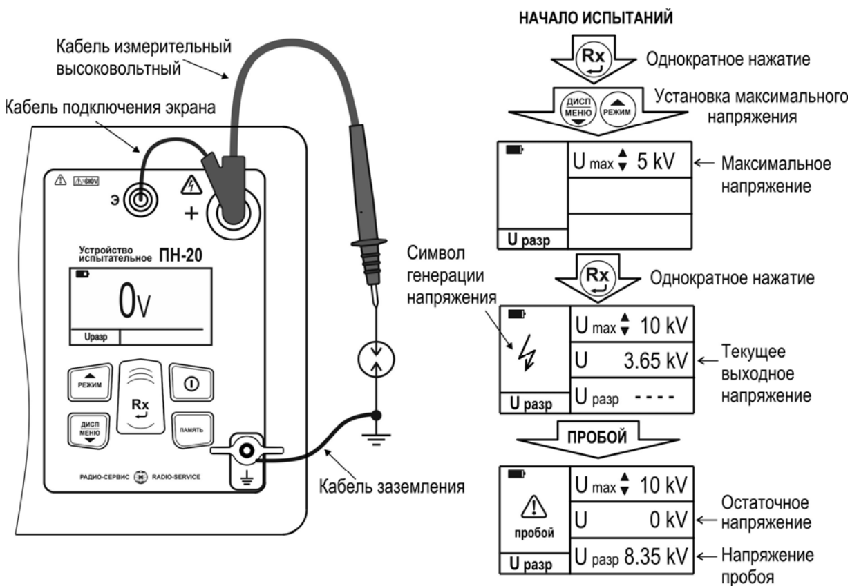
Рисунок 8 - Проверка напряжения пробоя разрядников
