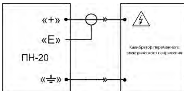
Рисунок 4 – Измерение переменного электрического напряжения частотой 50 Гц
