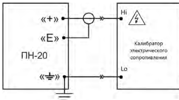
Рисунок 3 – Схема соединения при измерении электрического сопротивления
