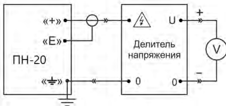
Рисунок 1 – Схема соединения при воспроизведении постоянного электрического напряжения
