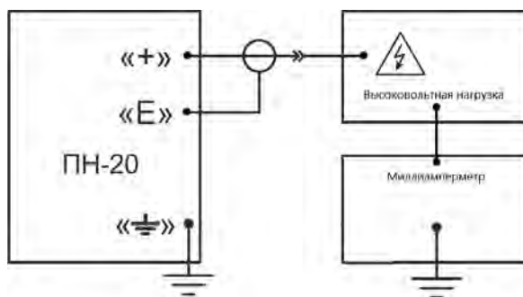
Рисунок 2 – Схема соединения при измерении силы постоянного электрического тока
