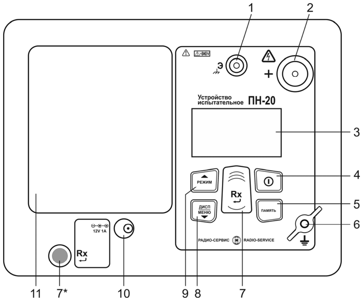
Рисунок 2 - Расположение разъёмов подключения и органов управления устройства
