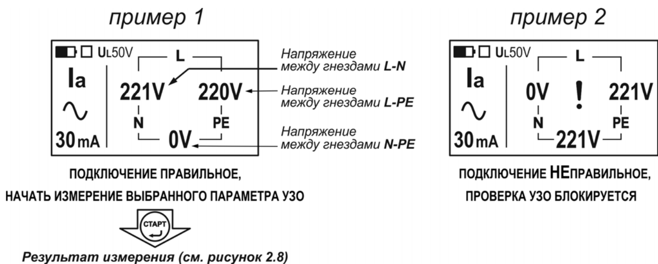
Рисунок 2.7 – Показания при измерении напряжения
