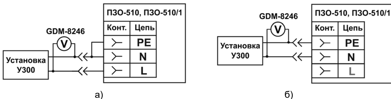
а) б) Рисунок 6.7.1 – Схемы проверки погрешности измерений напряжения переменного тока
